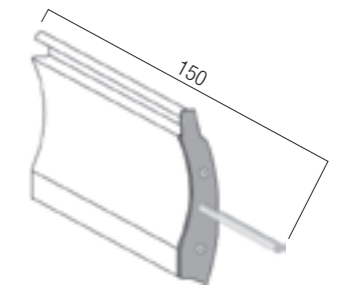
Caten. intermedio di sicurezza per stecca CATSTE000M 150 mm
